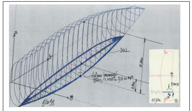
Carène chavirée à 90°
